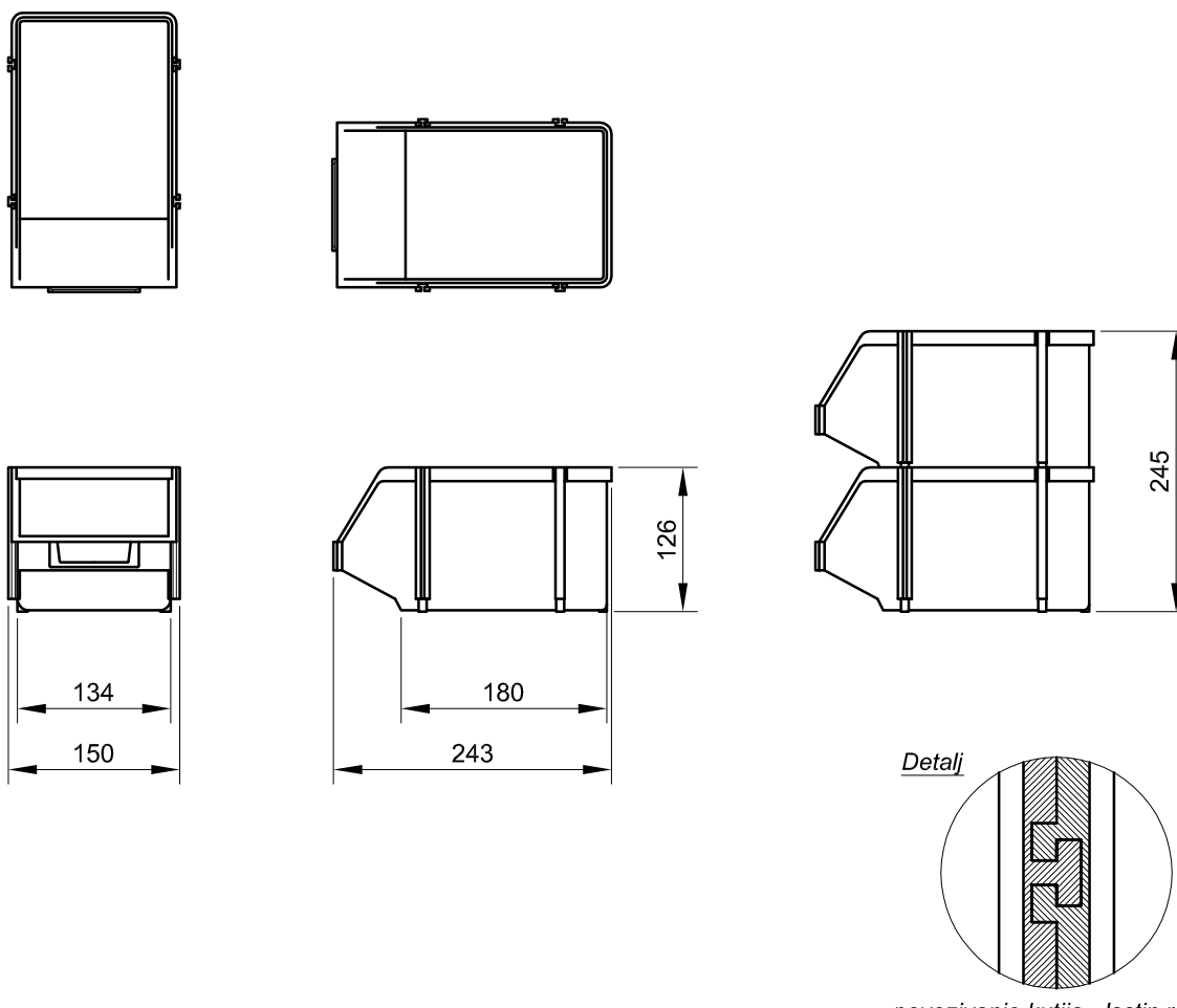
povezivanje kutija - lastin rep na bočnim stranicama kutije
